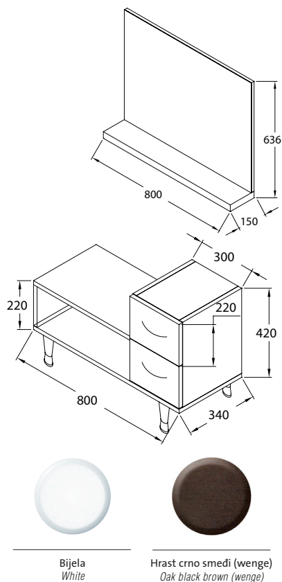
Kupaonski ormarić stajajući s nožicama, 2 ladice, polica s ogledalom/ Bathroom standing cabinet with legs, 2 drawers, shelf with mirror
